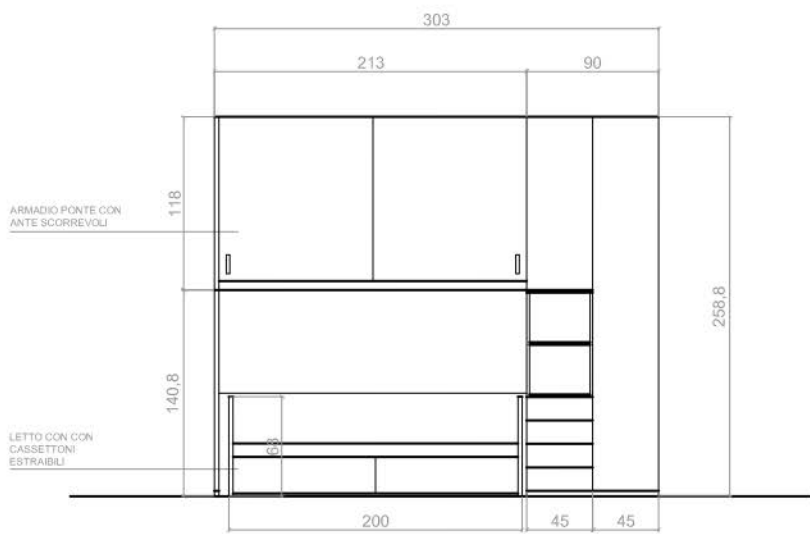
VISTA FRONTALE
