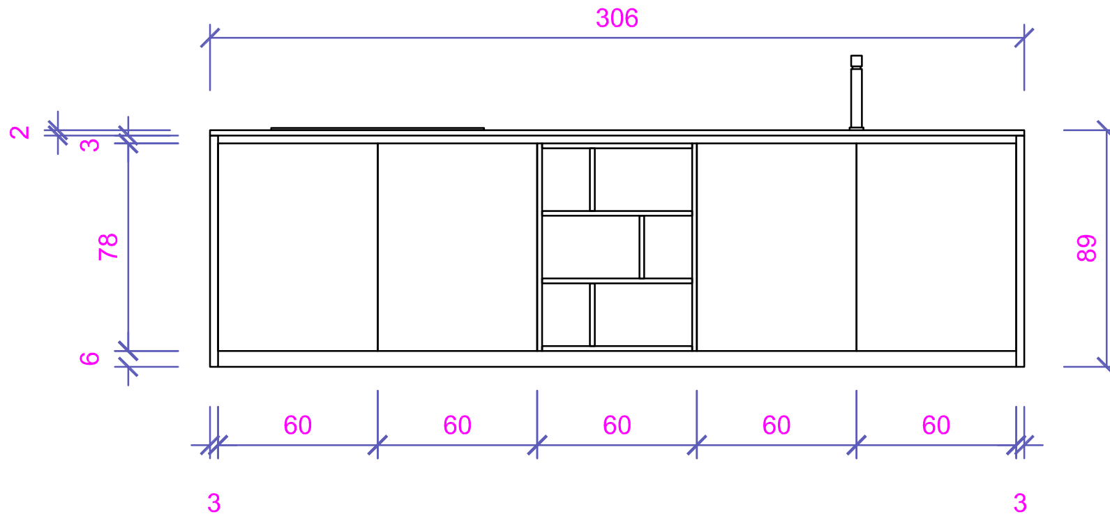
PROSPETTO "C"
