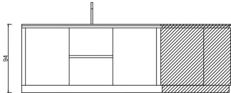
PROSPETTO A
