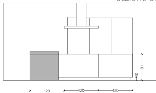
sezione CC
