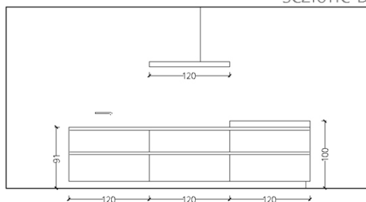
sezione BB
