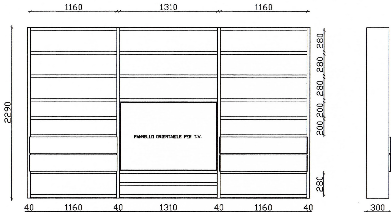
SEZIONE FRONTALE
