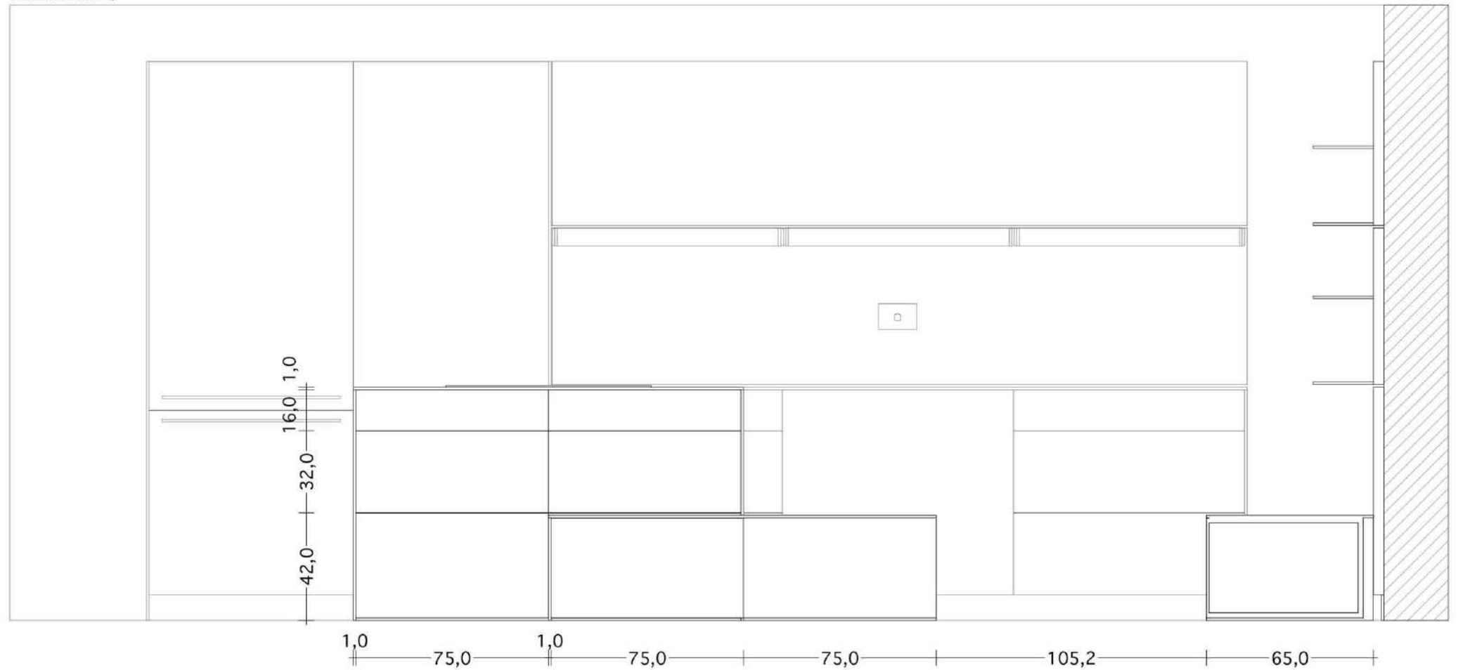
ELEVATION 5
