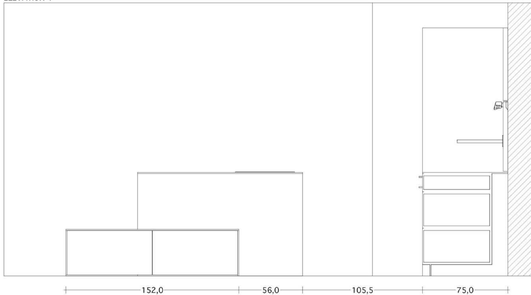
ELEVATION 4
