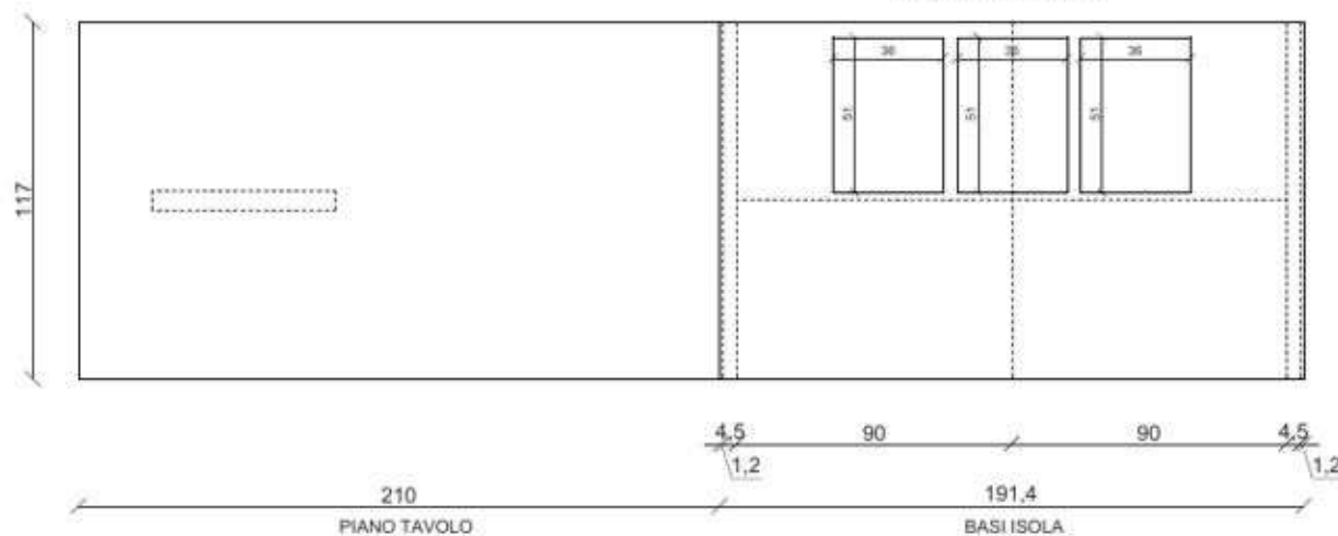
PROSPETTO C
