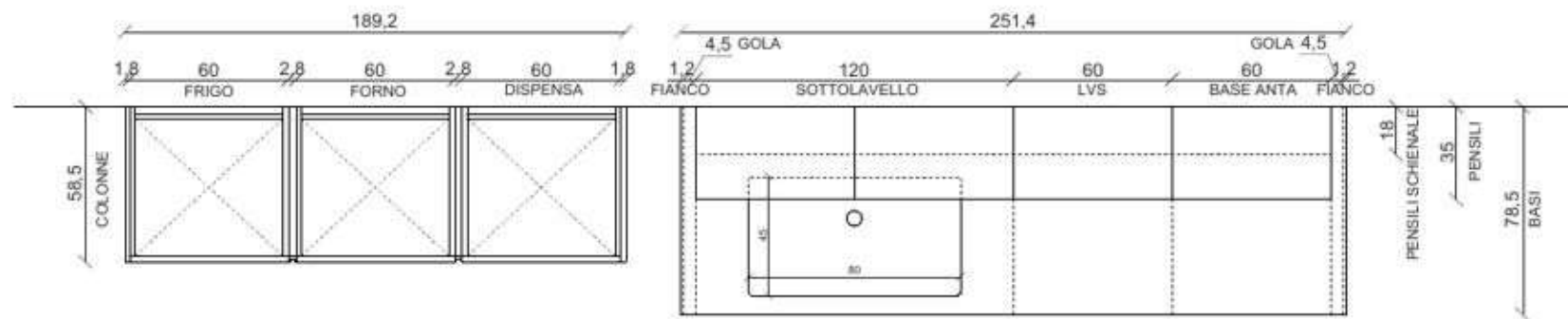
PROSPETTO A
