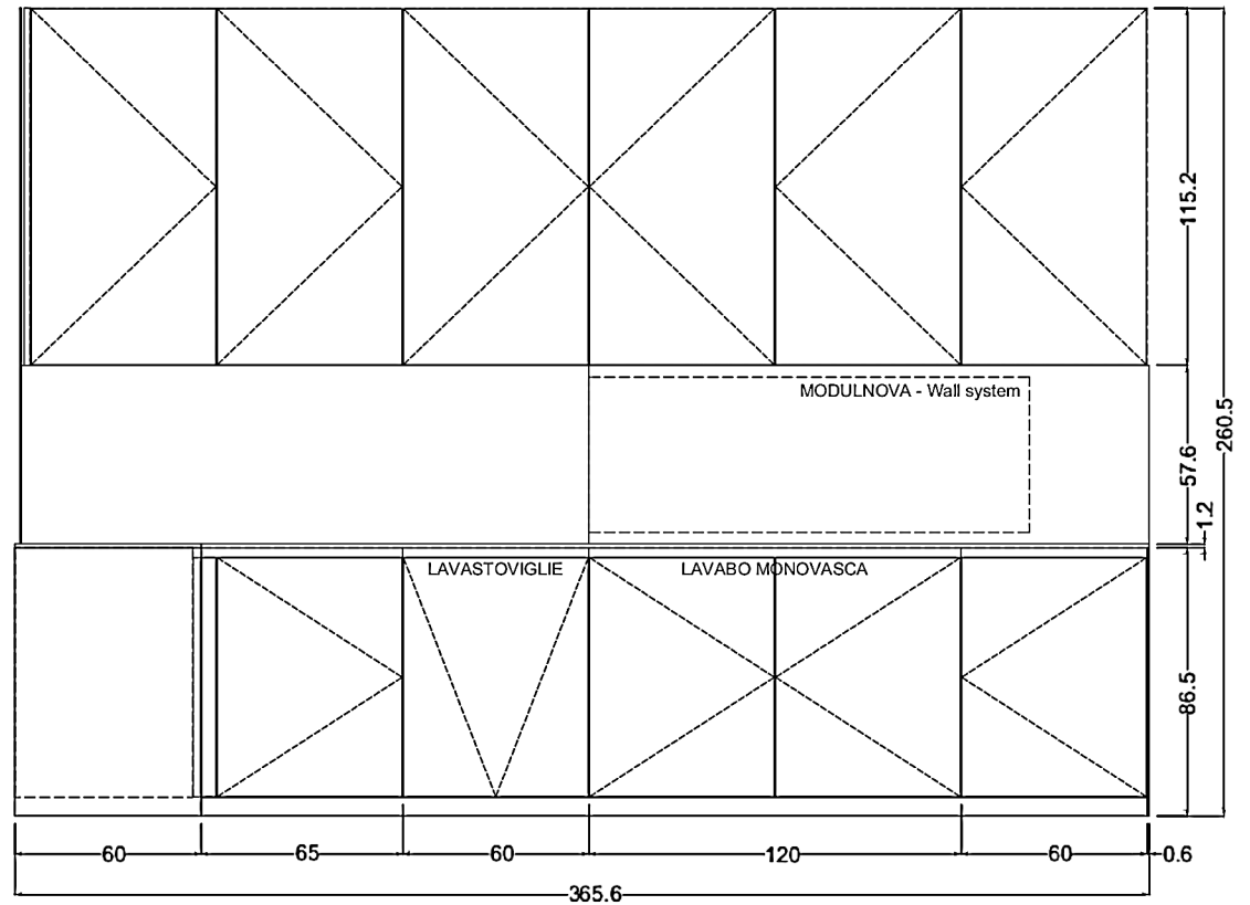
PROSPETTO FRONTALE - LATO LAVABO
