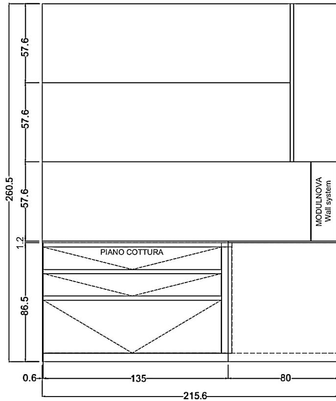
PROSPETTO FRONTALE - LATO PIANO COTTURA
