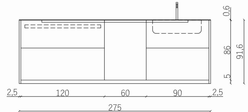
COMPOSIZIONE ISOLA VISTA IN PROSPETTO
