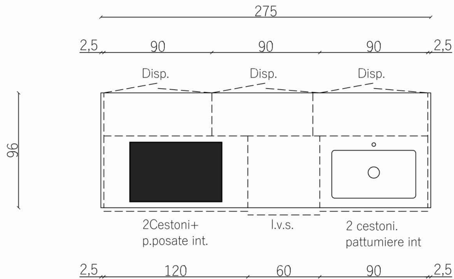
COMPOSIZIONE ISOLA VISTA IN PIANTA
