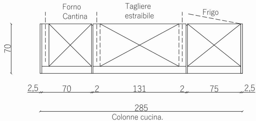
COMPOSIZIONE COLONNE VISTA IN PIANTA
