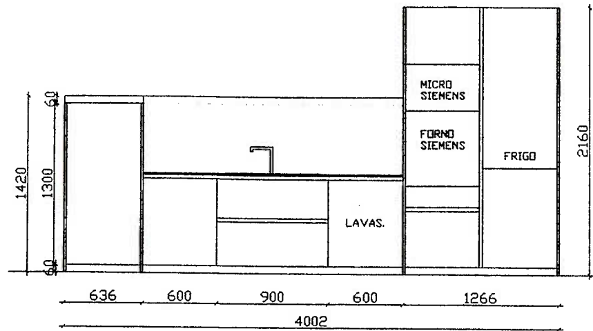
SEZIONE FRONTALE
