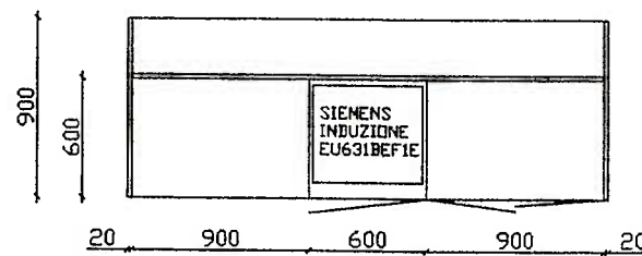
PIANTA ISOLA
