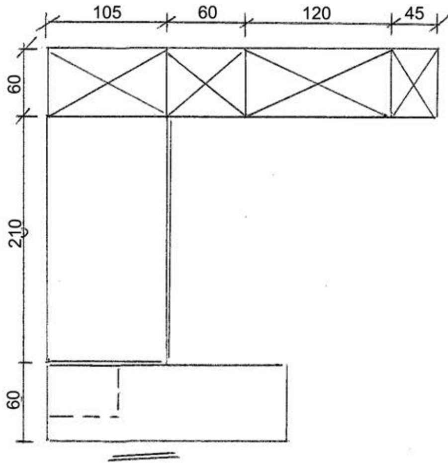
PIANTA
