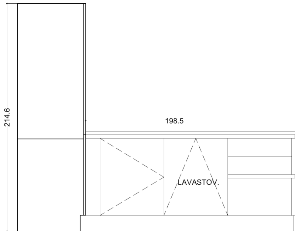
PROSPETTO B
