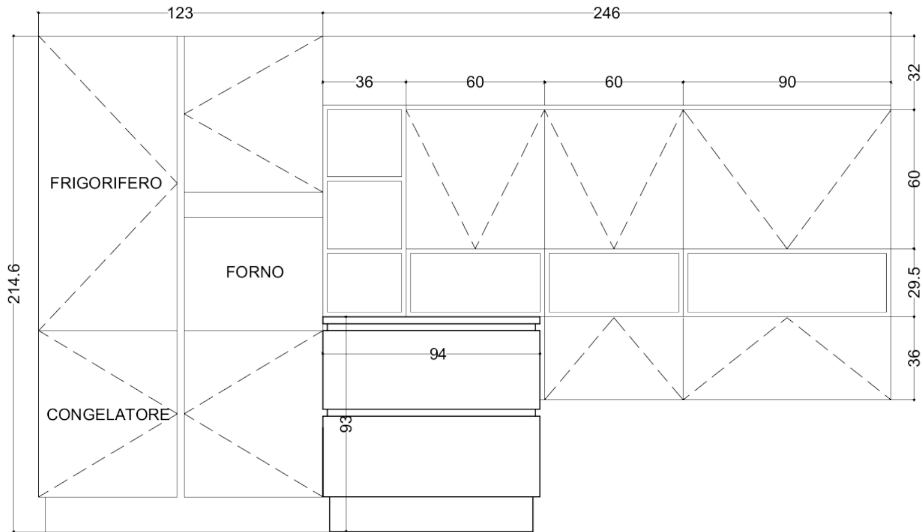
PROSPETTO A
