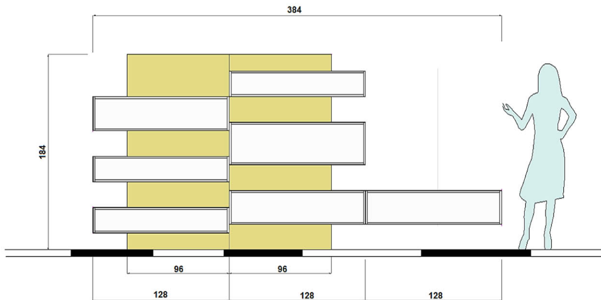
PROSPETTO
