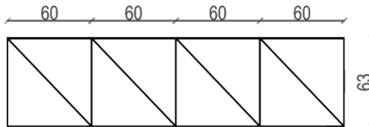
prospetto colonne
