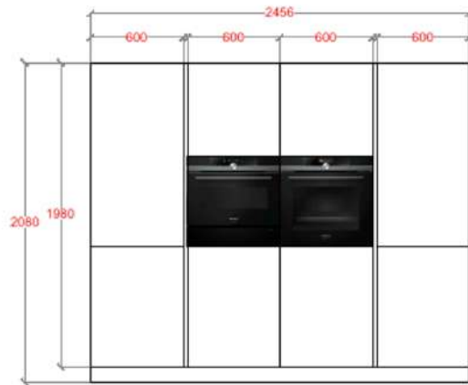
ALEA PRO Poliform Kitchen PROSPETTO COLONNE
