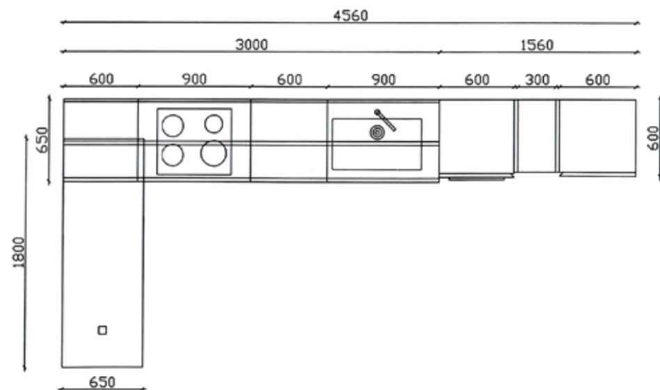
PIANTA CUCINA
