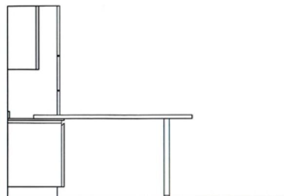
SEZIONE LATERALE CUCINA (TOP PENISOLA IN APPOGGIO SPOSTABILE)
