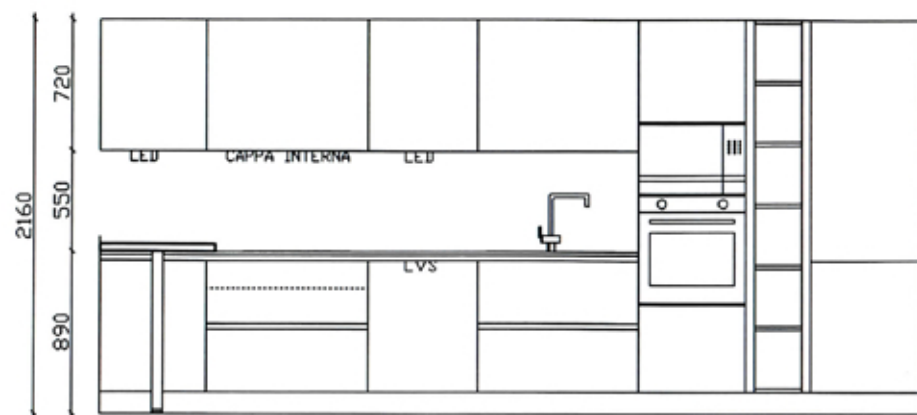
SEZIONE FRONTALE CUCINA CON PIANO PENISOLA IN APPOGGIO SPOSTABILE
