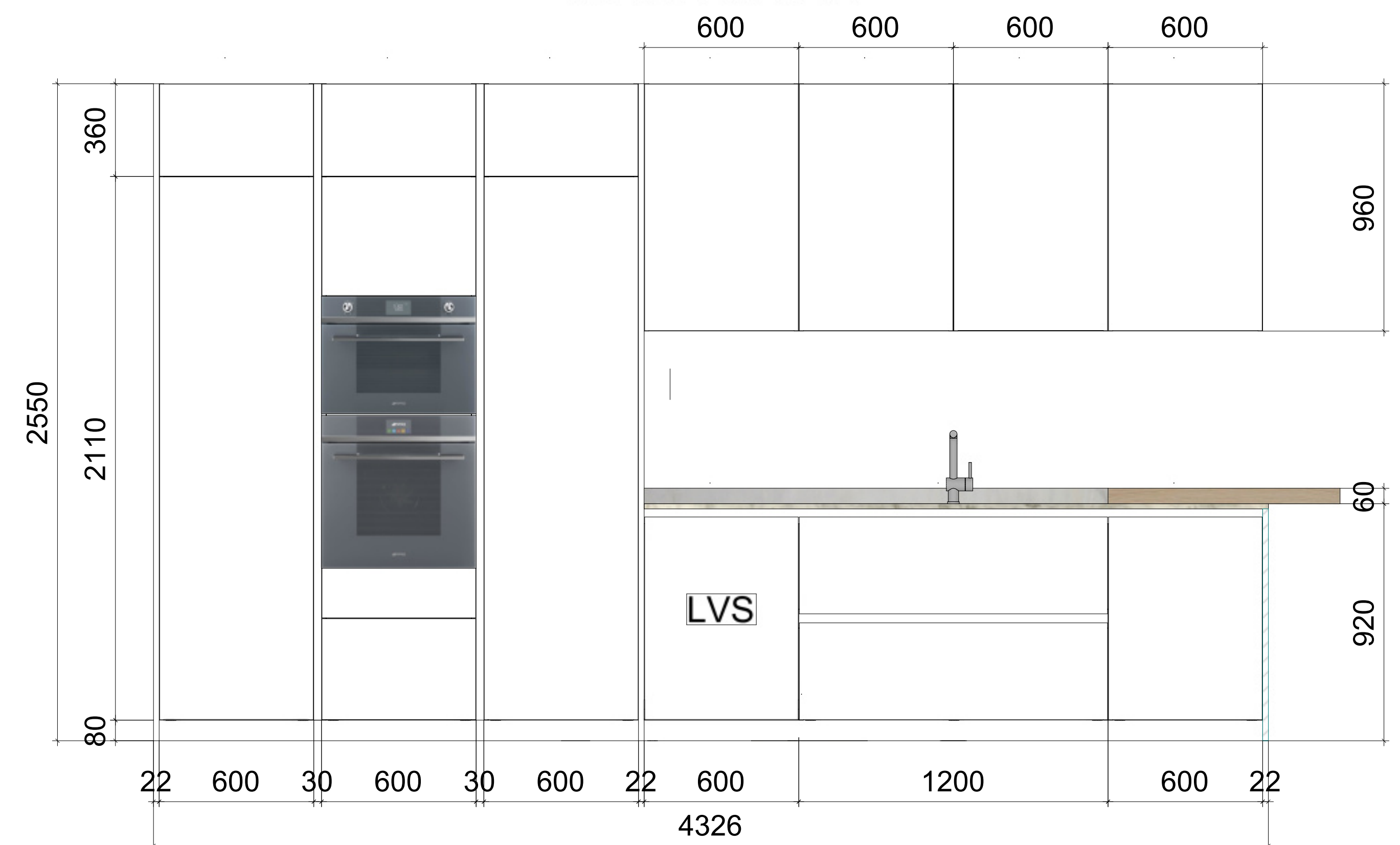
VISTA PARETE A
