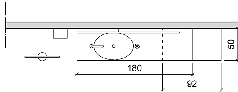
Prospetto A
