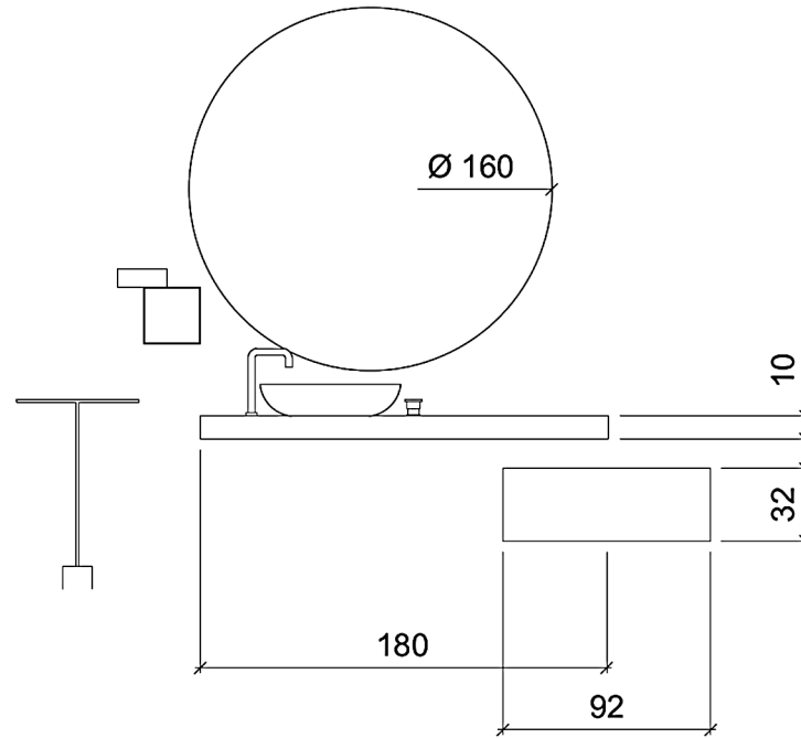
Prospetto A
