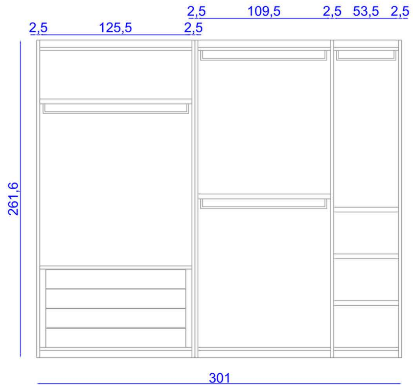
FRONTALE INTERNO ARMADIO
