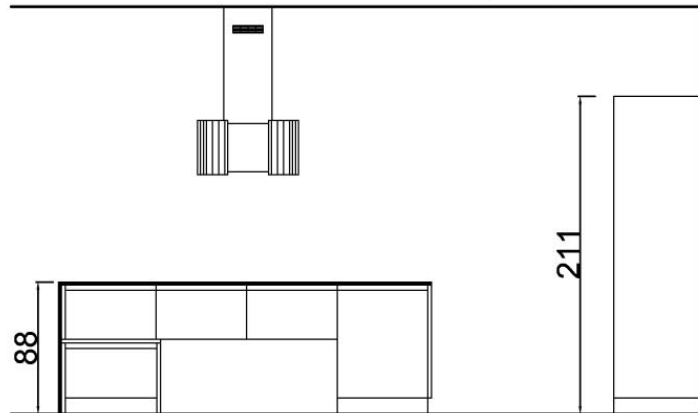
prospetto AA
