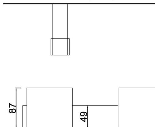
prospetto DD
