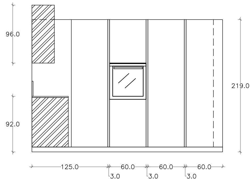
PROSPETTO COLONNE
