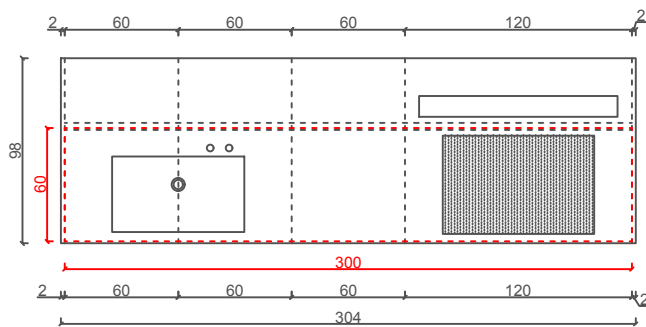
PIANTA ISOLA
