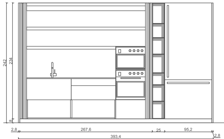
PROSPETTO COLONNE
