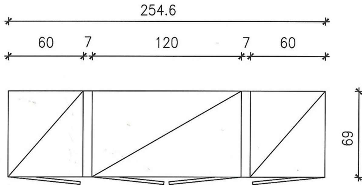
PIANTA PARETE ATTREZZATA
