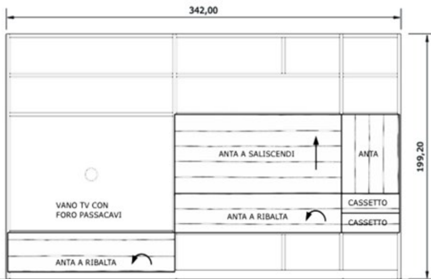
VISTA FRONTALE CON ANTE
