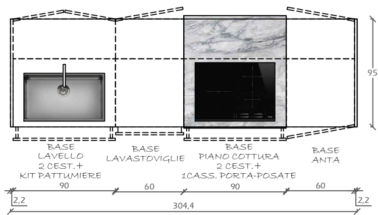
PIANTA BASI
