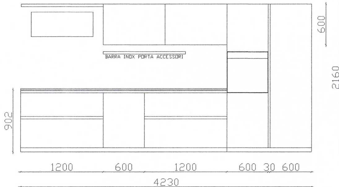
SEZIONE FRONTALE CUCINA
