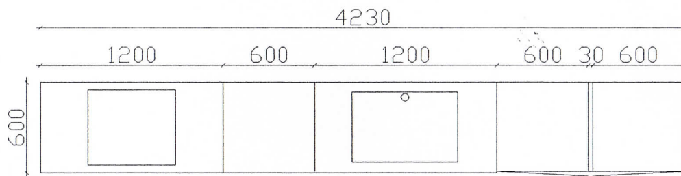
PIANTA CUCINA
