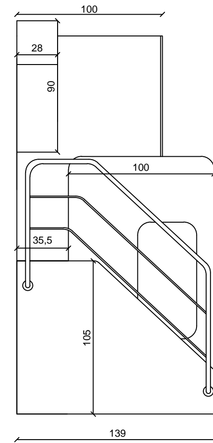
PROSPETTO CAMERETTA B
