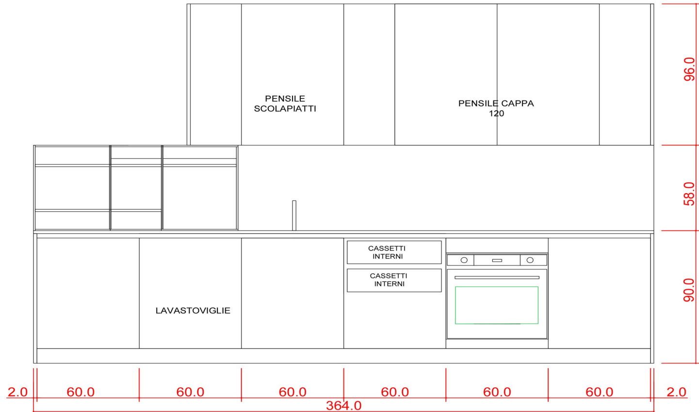
PROSPETTO
