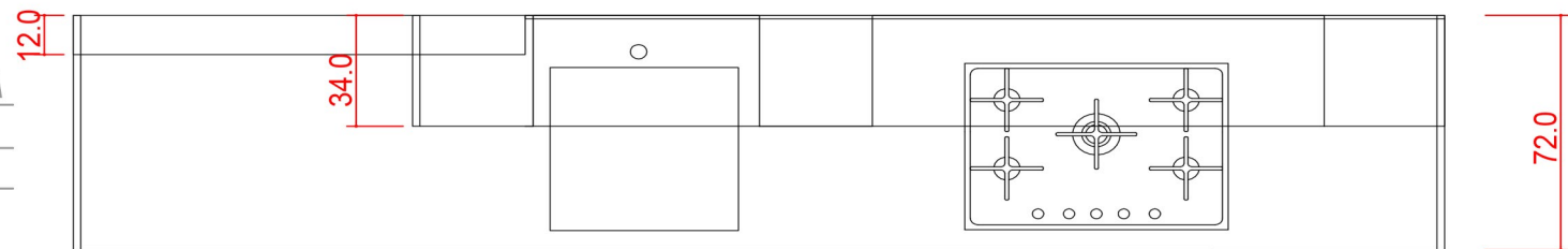
PLANIMETRIA
