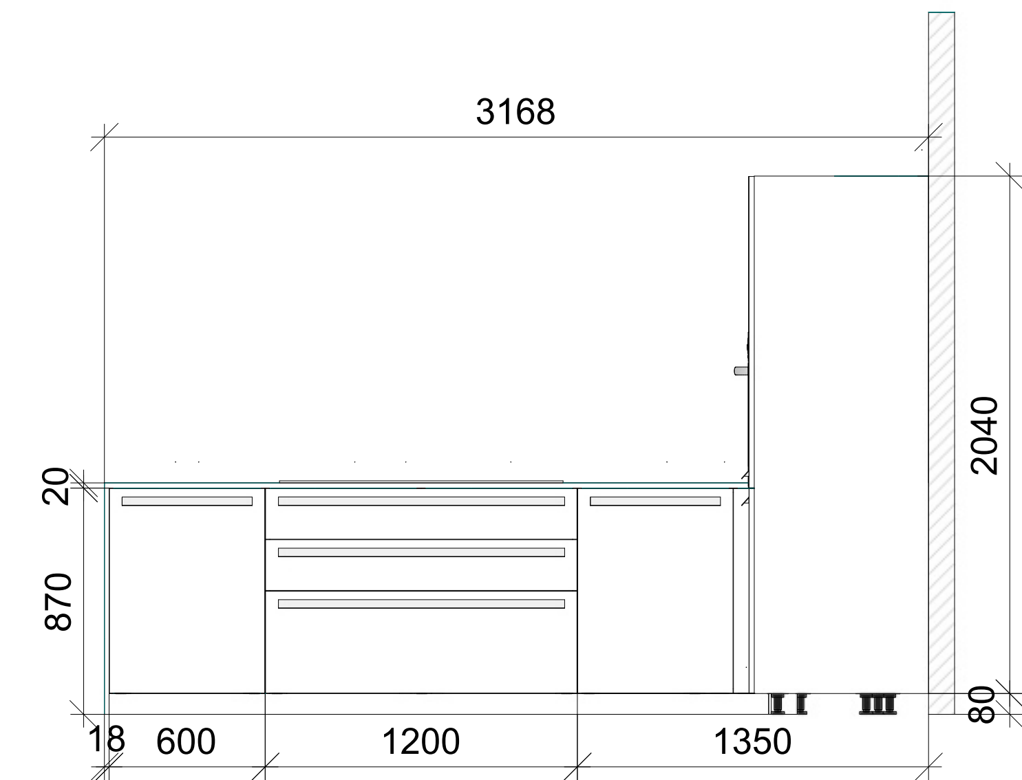
VISTA PARETE B
