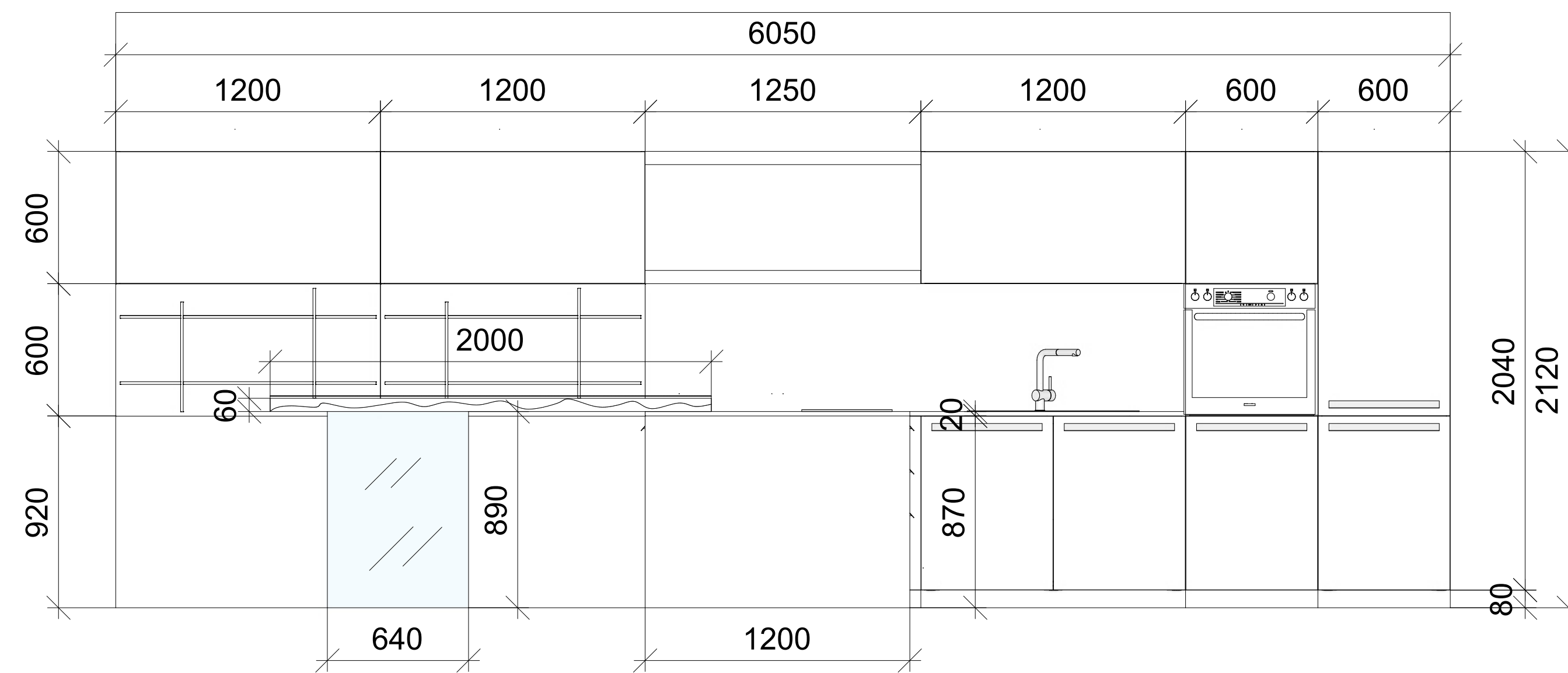
VISTA PARETE A
