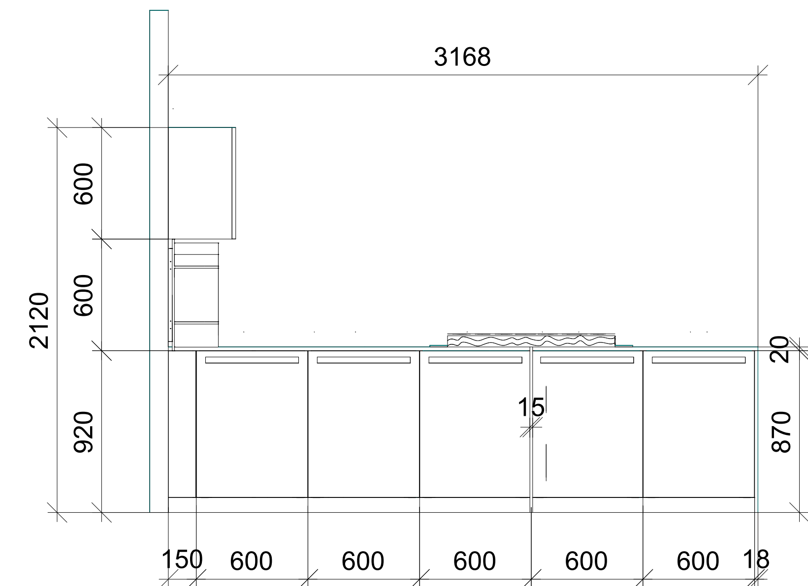
VISTA PARETE C
