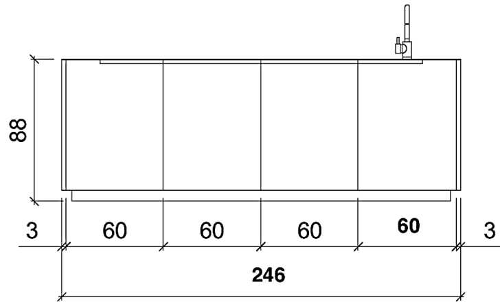
Prospecto A
