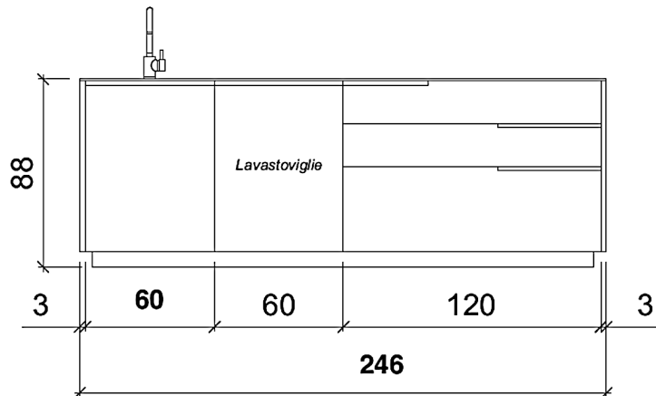
Prospecto B
