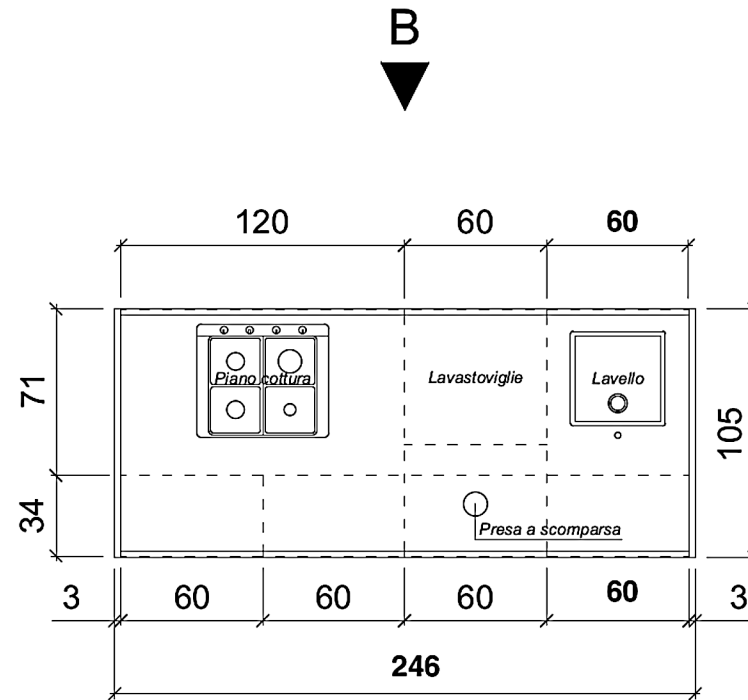
Vista dall'alto
