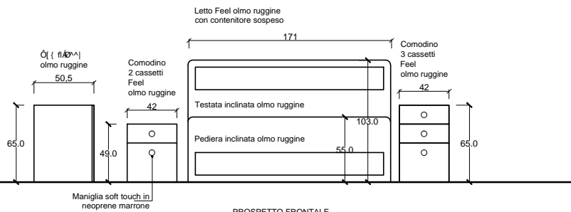
PROSPETTO FRONTALE
