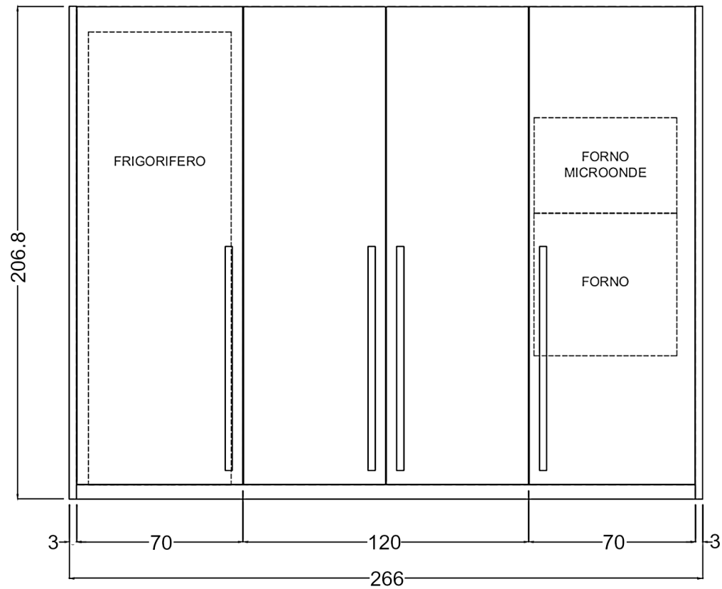
PROSPETTO FRONTALE
