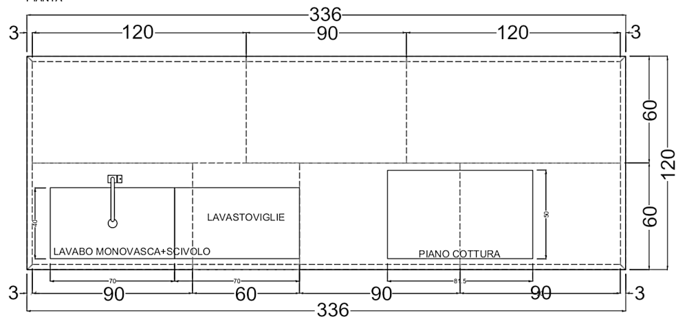
PIANTA
