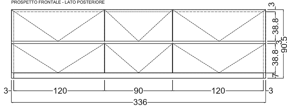
PROSPETTO FRONTALE - LATO POSTERIORE
