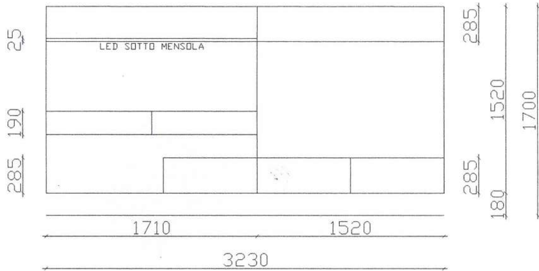
SEZIONE FRONTALE SOGGIORNO
