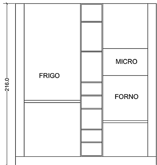
PROSPETTO COLONNE
