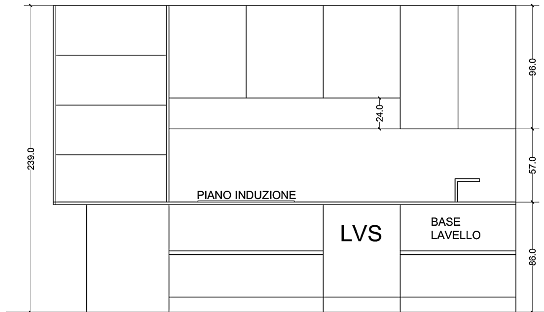
PROSPETTO CUCINA
