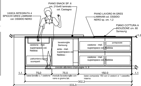
PROSPETTO LATO A
