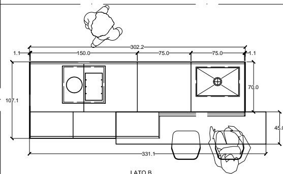
LATO B
