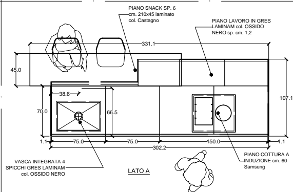
PROSPETTO LATO A
